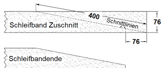
Abb. 6-6: Schleifbandzuschchnitt
