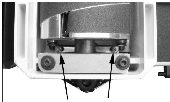
Figure 8-4: vis de réglage de tension
